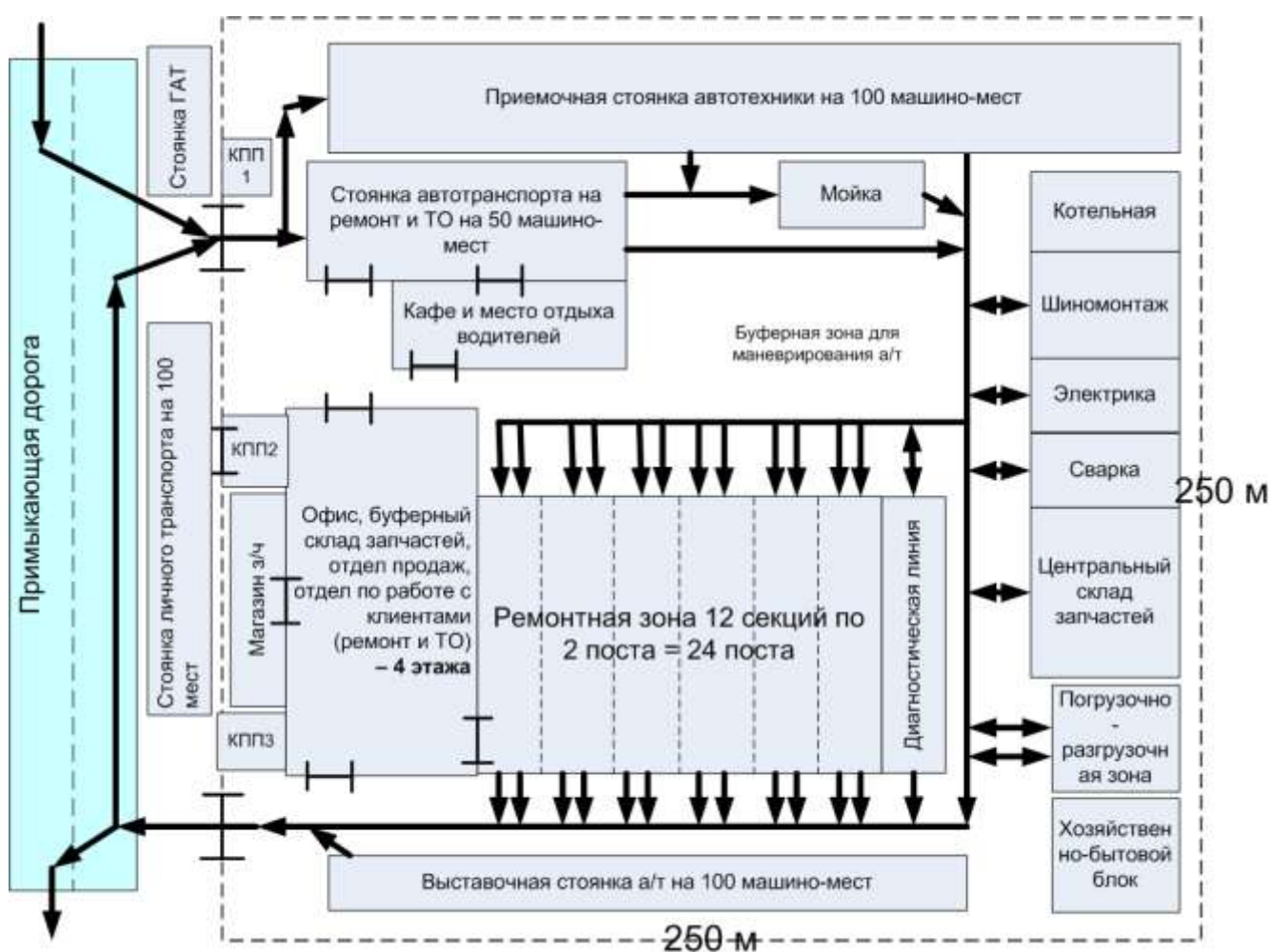
Рис. 4.1. Примерная планировка РЦ КАМАЗ
